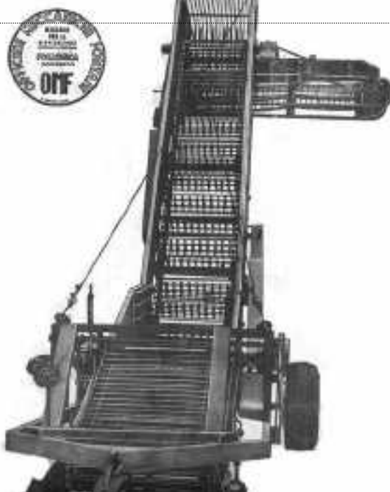
Caricatore da bietole (Officine Fontani di Follonica - Gr)
