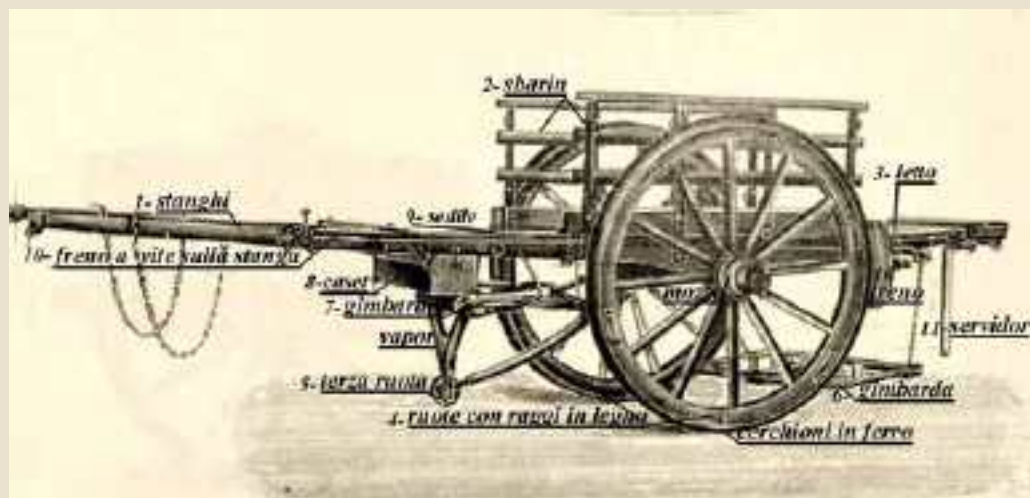
Carro a due ruote: componenti principali
