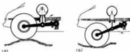
SCHEMA SOSPENSIONE IDROPNEUMATICA
