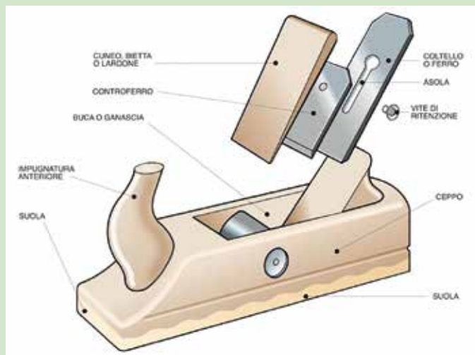
Struttura della pialla a mano
