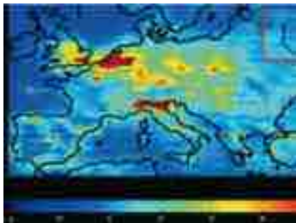
Mappa di NO 2 determinata da satellite: si notano le aree più compromesse, la Pianura Padana e i Paesi Bassi
